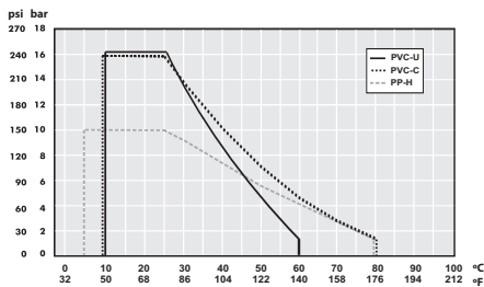
Druck-Temperatur-Diagramm (G 3.1)
