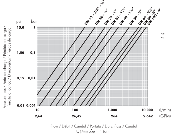
Druckverlus-Diagramm (G 3.3)
