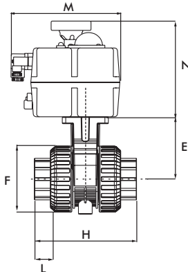
Dimensiones de acople de actuador (T4.2)
